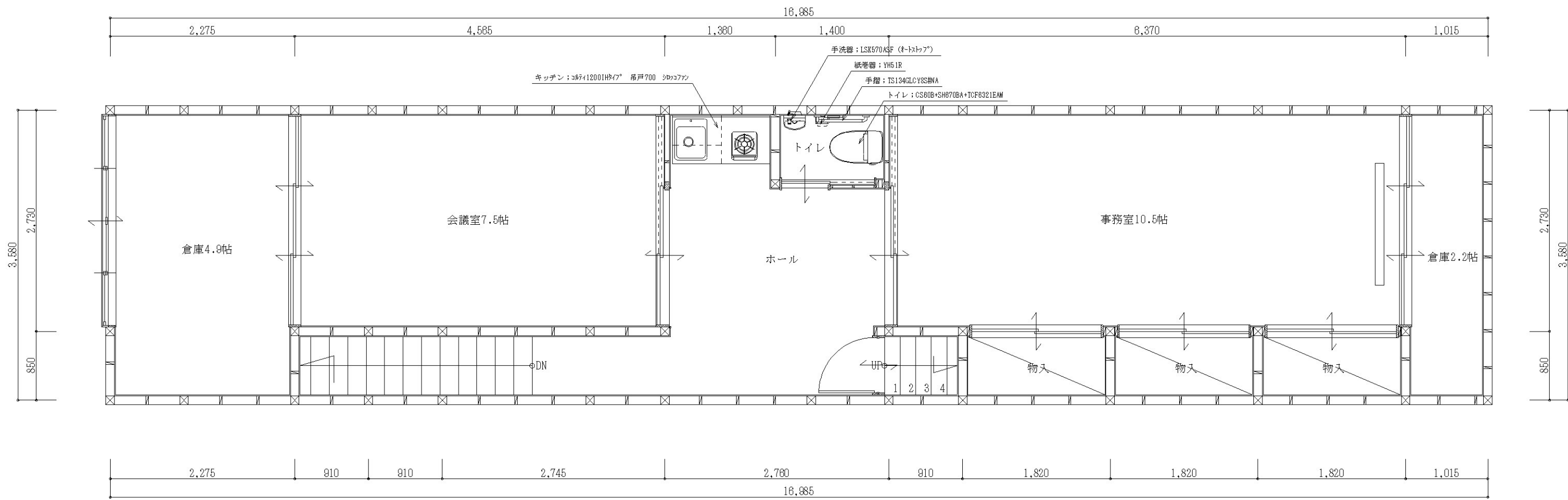
2階 平面詳細図 S:1/50
