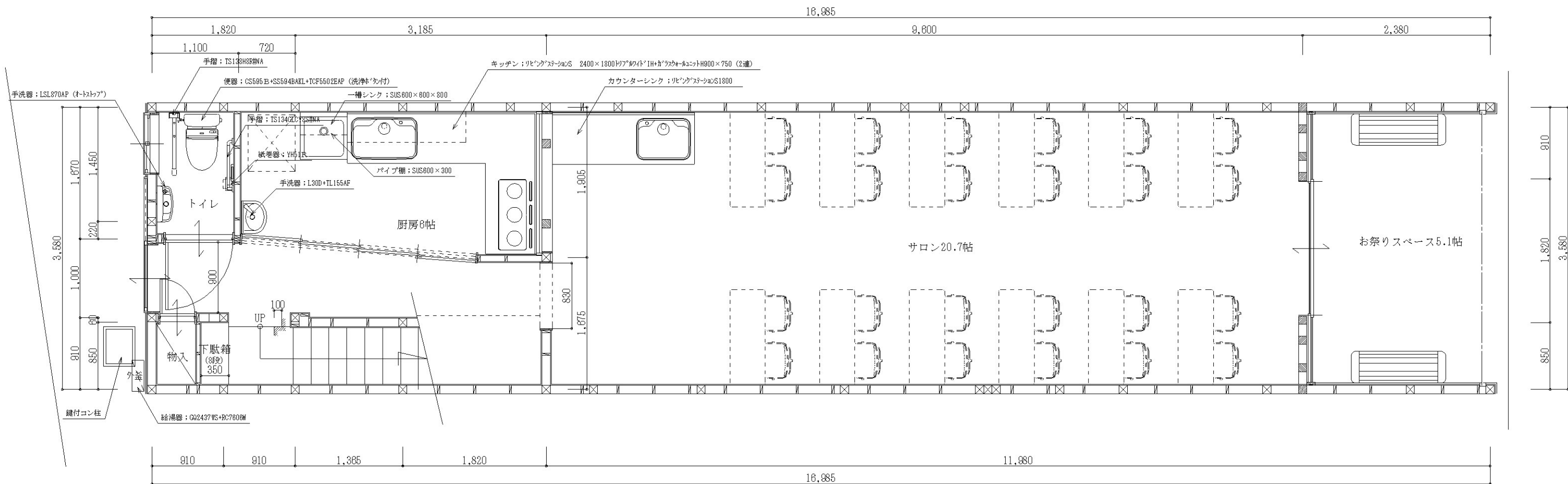
1階 平面詳細図 S:1/50
